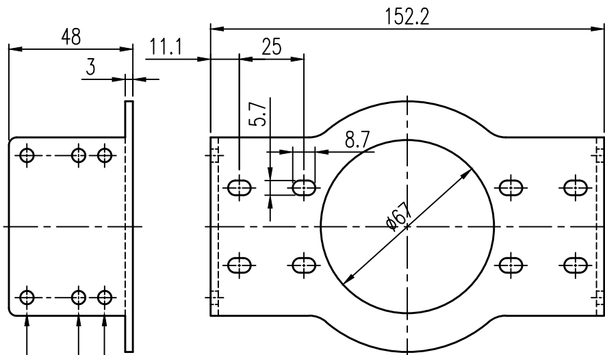
ACTUATOR BRACKET
