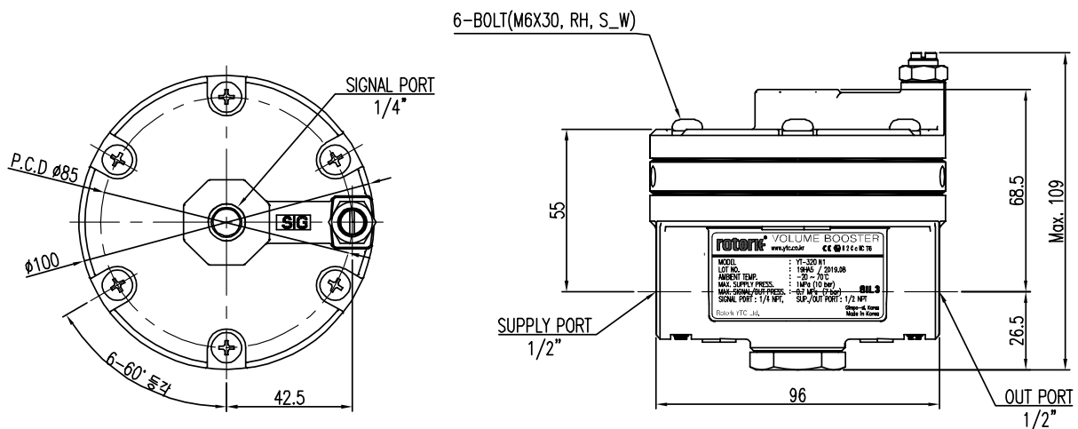
Fig. 2-7: YT-320 / 325 dimension
