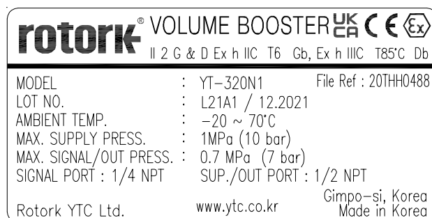
Fig. L-7: YT-320 (UKEX,ATEX)
