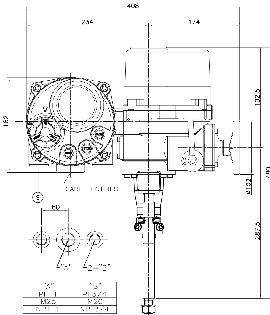
CABLE ENTRIES
