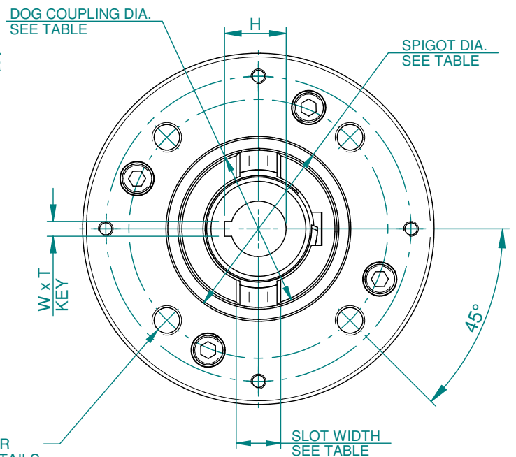
F14/FA14 NON THRUST BASE (B1, B3 & B4)
