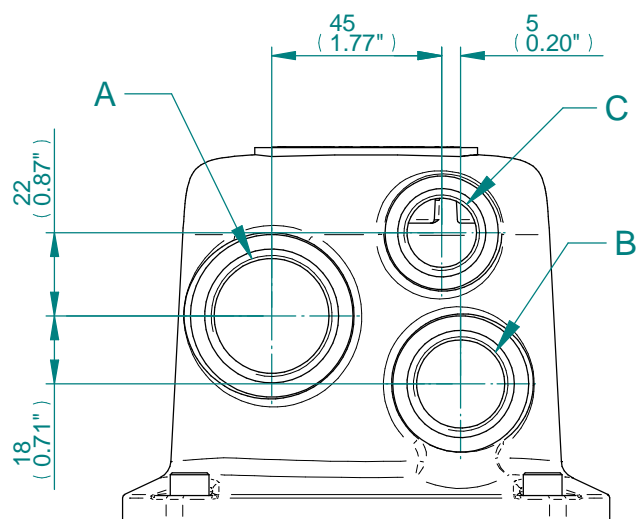
CONDUIT ENTRIES
