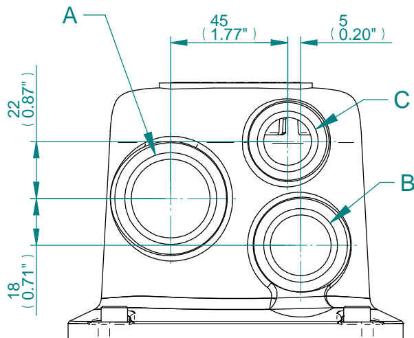
CONDUIT ENTRIES
